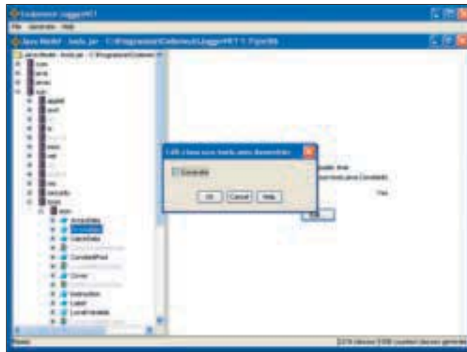
Abbildung 2 JuggerNET Code-Generator.
